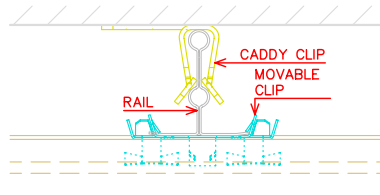
HORIZ. SECTIONS
